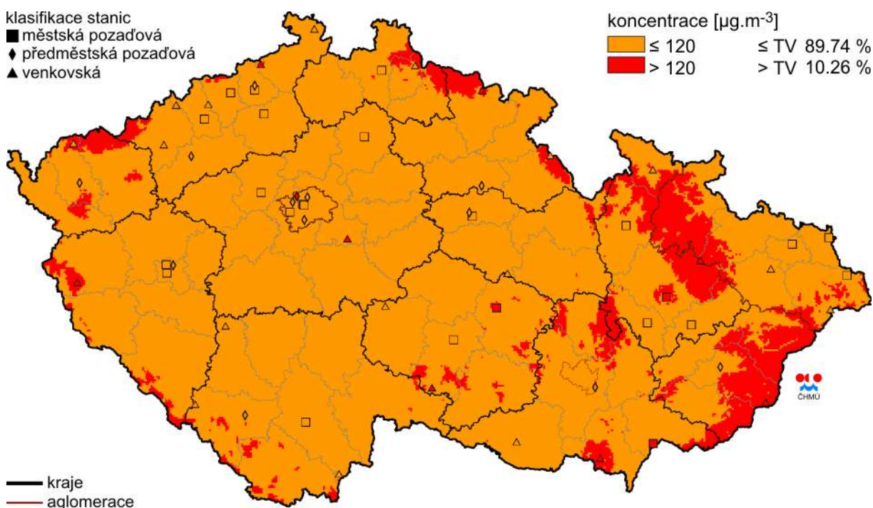
Obr. 33. Pole 26. nejvyššího maximálního denního 8hodinového klouzavého průměru koncentrace ozonu v průměru za 3 roky, 2008–2010 (zdroj ČHMÚ)
