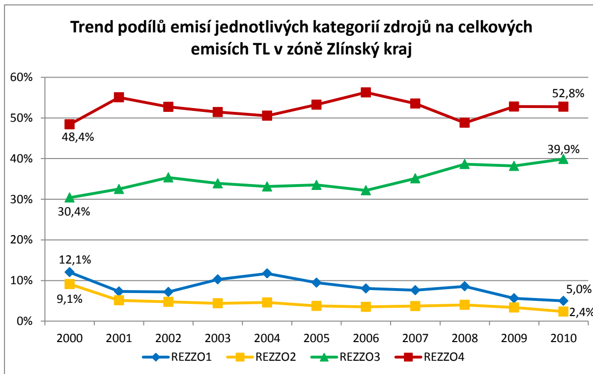
Obr. 44. Trend podílů kategorií zdrojů na celkových emisích TL
