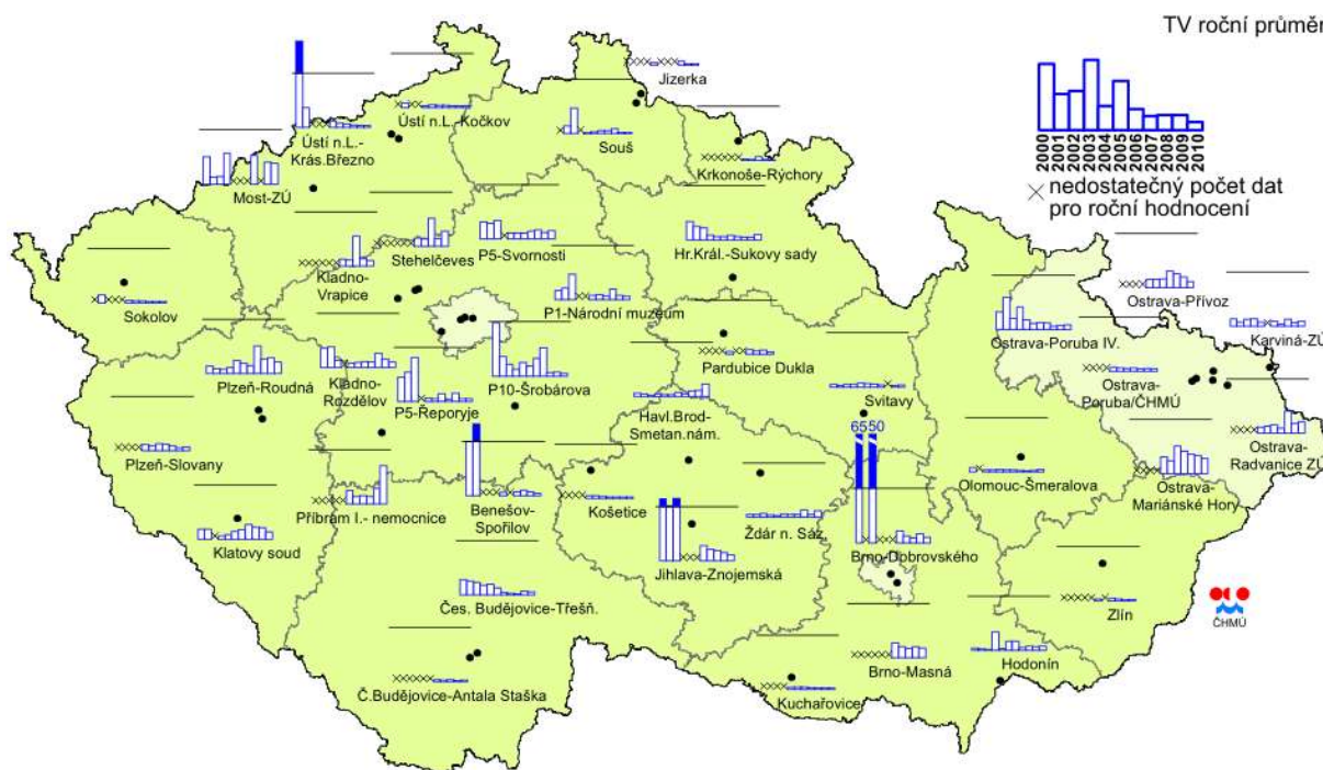
Obr. 39. Stanice s nejvyššími ročními průměrnými koncentracemi niklu v ovzduší v roce 2010 (zdroj ČHMÚ)
