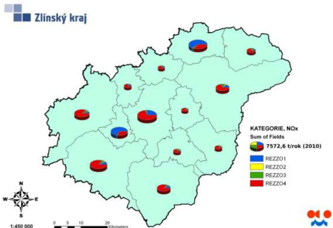
Obr. 49. Mapa emisí NO x dle kategorií zdrojů v jednotlivých ORP, rok 2010
