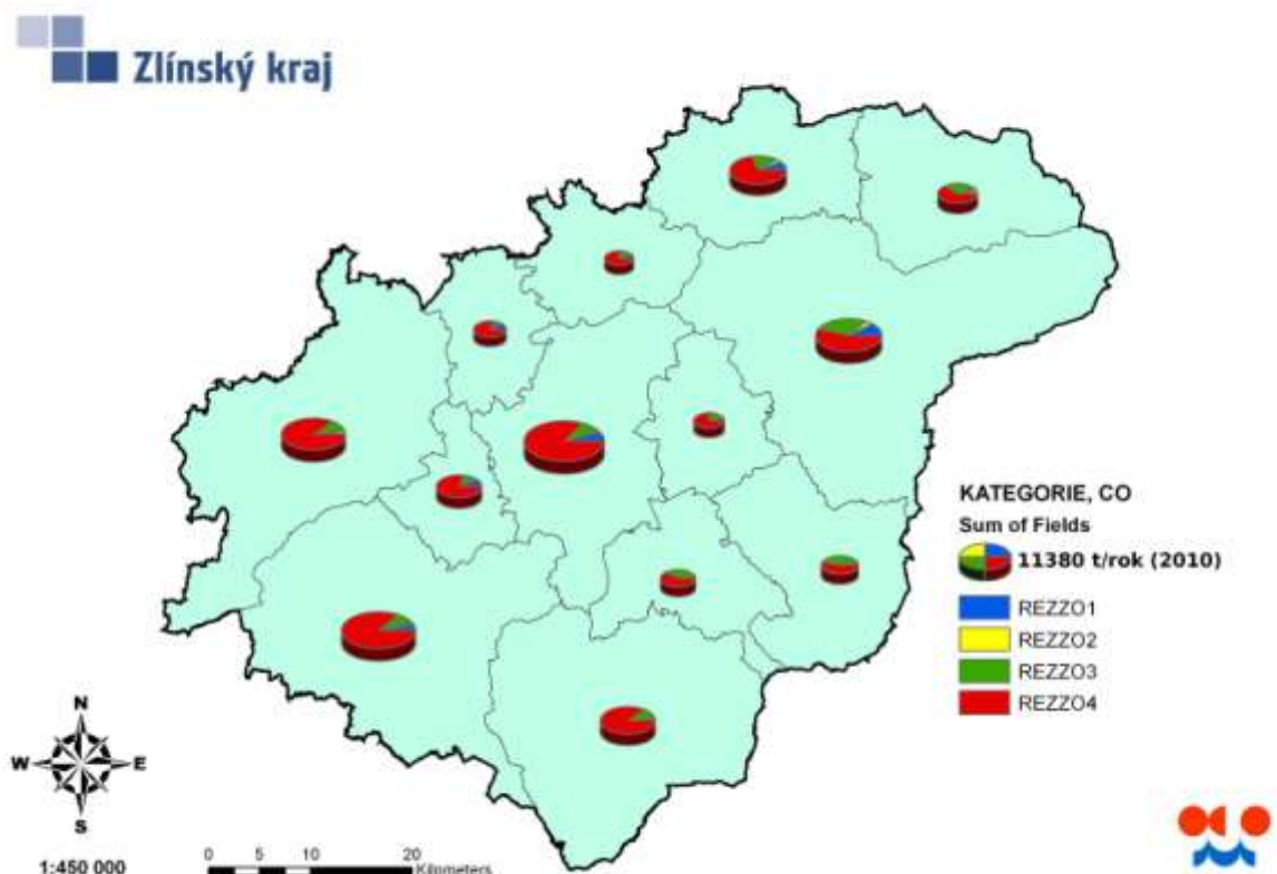
Obr. 51. Mapa emisí CO dle kategorií zdrojů v jednotlivých ORP, rok 2010
