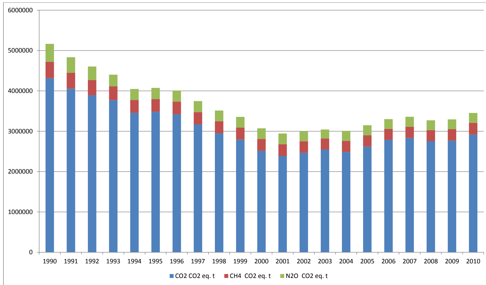
Obr. 56. Emise skleníkových plynů – podíl jednotlivých plynů, Zlínský kraj 1990 - 2010
