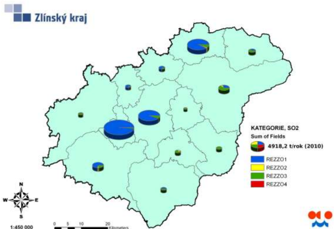
Obr. 47. Mapa emisí SO 2 dle kategorií zdrojů v jednotlivých ORP, rok 2010
